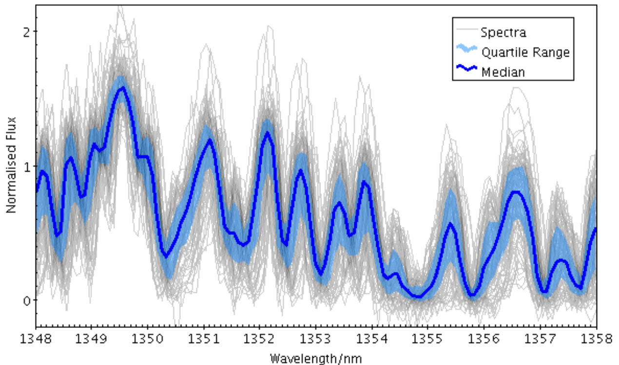
Example ArrayQuantile plot
